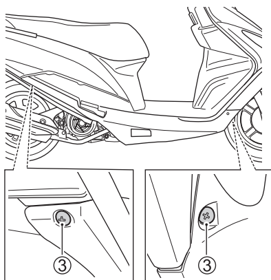
右视图
